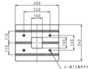
ボルスタ寸法図
