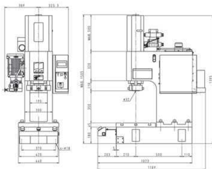
HYP100 P 寸法図
