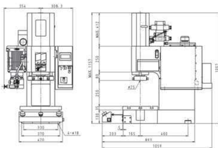
HYP50 HP 寸法図
