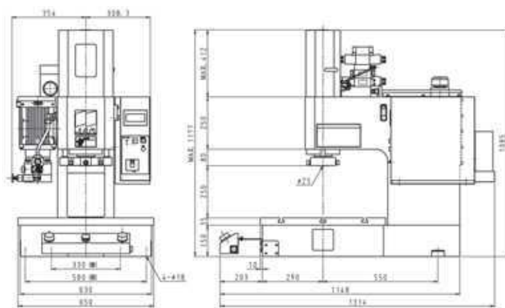
HYP50 DP 寸法図
