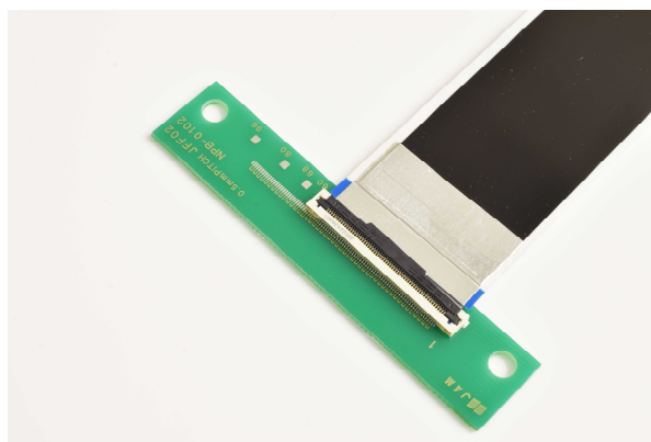
FFC/FPC仮保持機構
