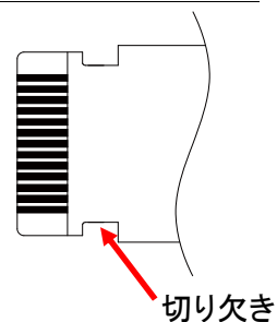
FFC/FPC仮保持機構
