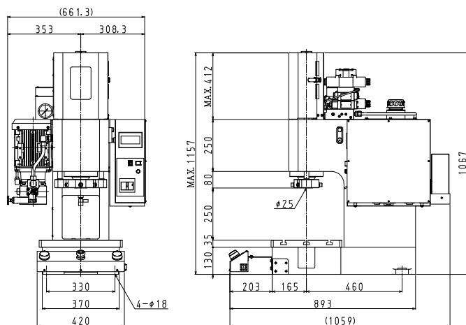
HYP50HP 寸法図
