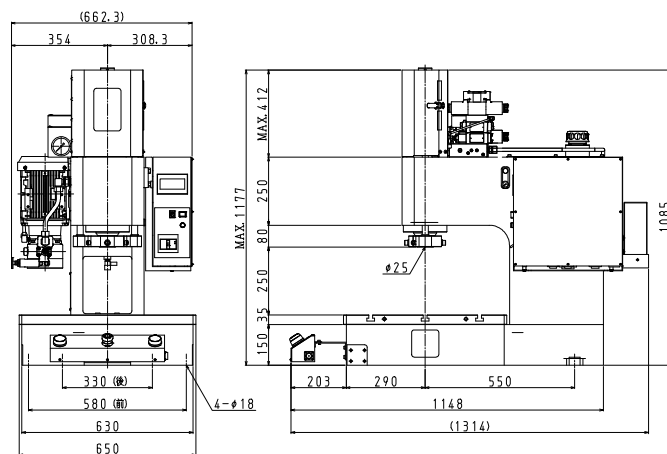
HYP50DP 寸法図
